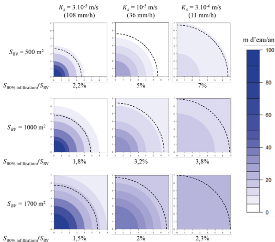
Figure 8.2 – Lamé d'eau infiltrée (exprimée en mètres d'eau par an) dans les différentes zones d'un espace de 50 m² sans exutoire, en fonction de la perméabilité du sol K_s et de la surface du bassin versant S_{BV} . La courbe en pointillés délimite la zone où s'infiltré 80% de la pluie totale.
