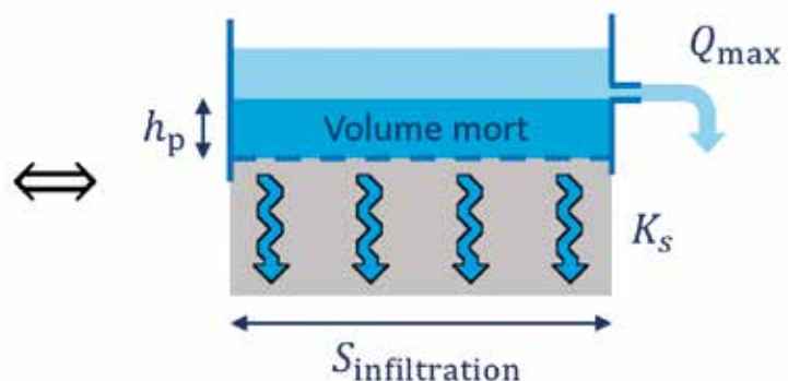
Figure 2.2 – Représentation simplifiée d'un dispositif de gestion à la source des eaux pluviales (© Portland Green Streets tour map, 2007).
